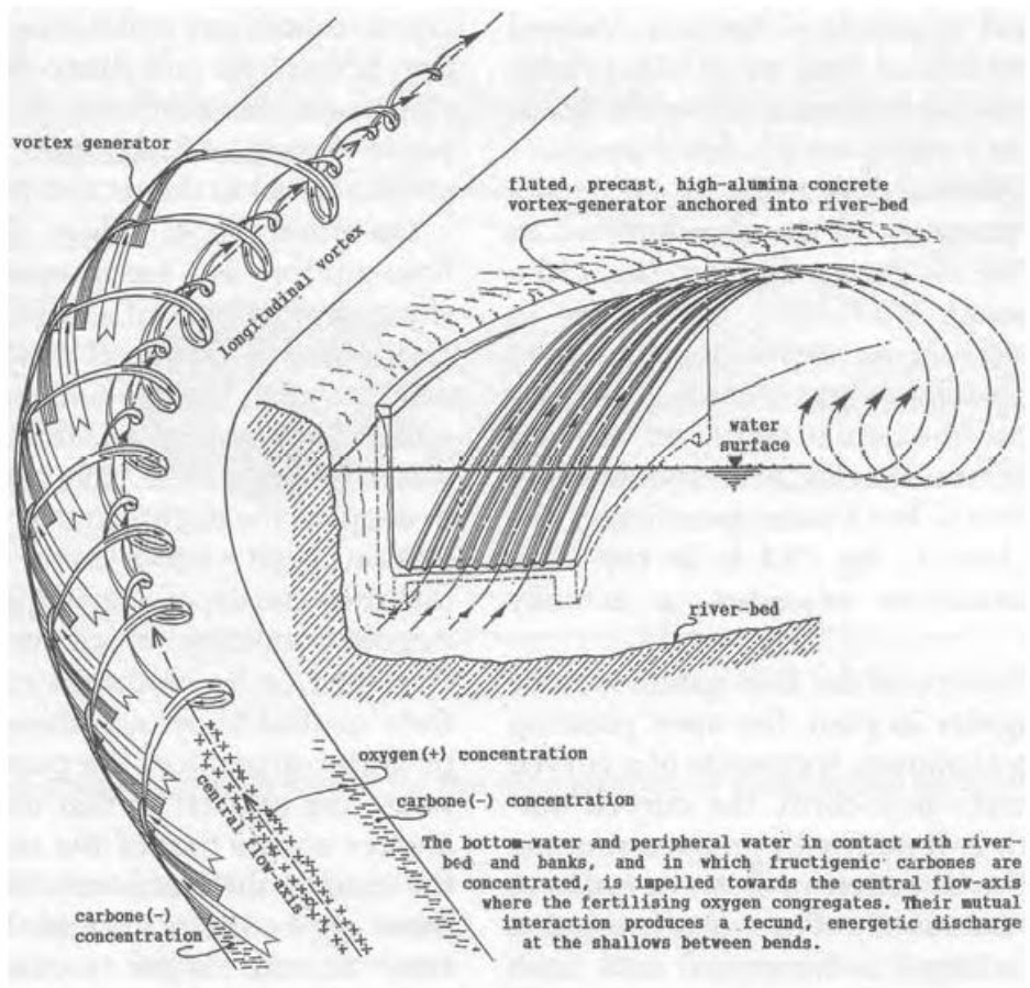
Fig. 13.4 Longitudinal vortex-generator
