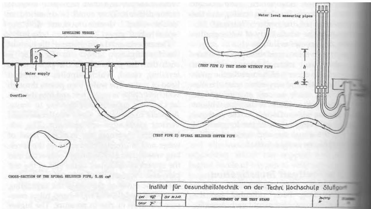
Рис. 14.6 в эксперименте со сферически-спиральной медной трубой, проф Попель
