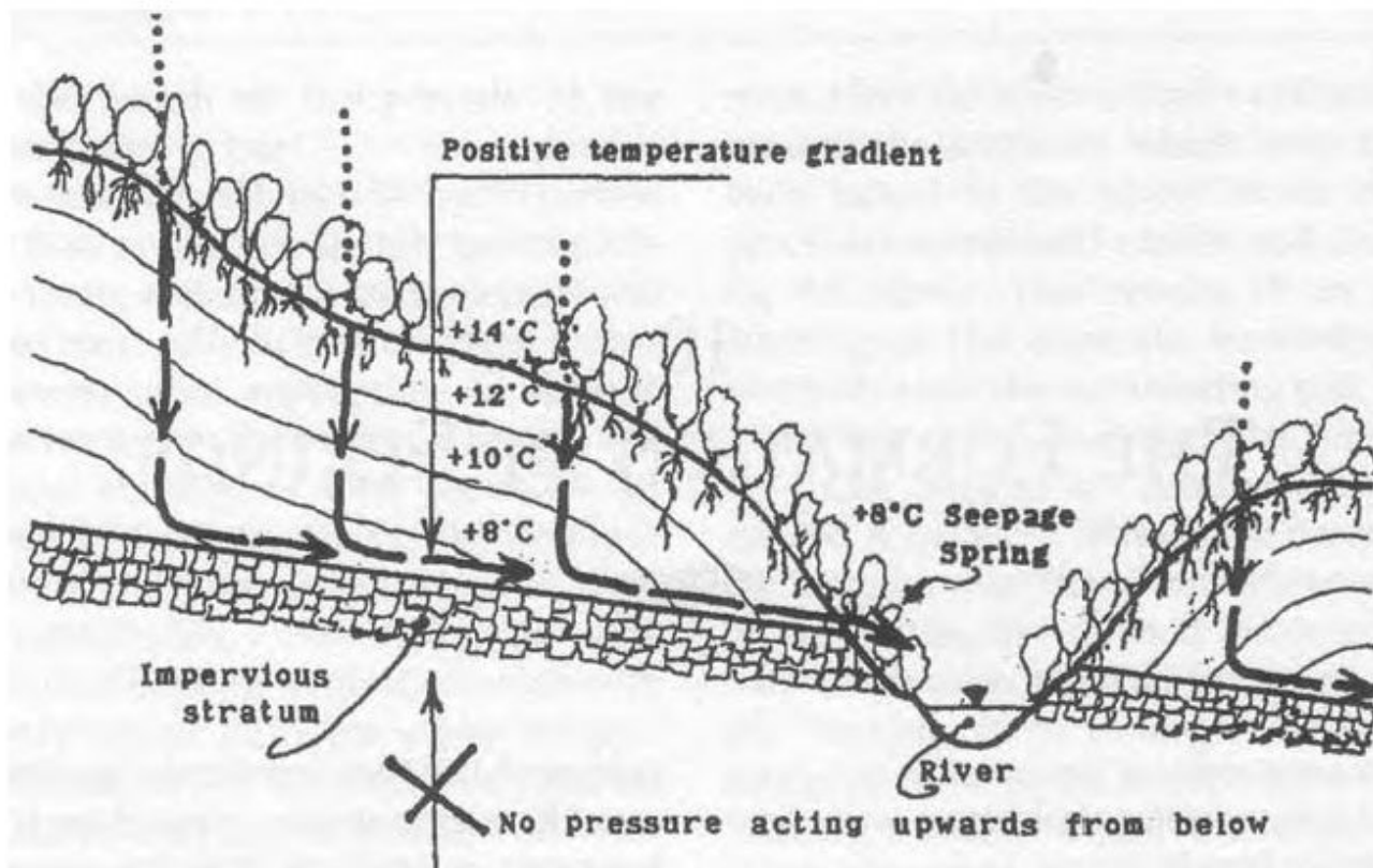
Рис. 10,1 Просачивание воды
