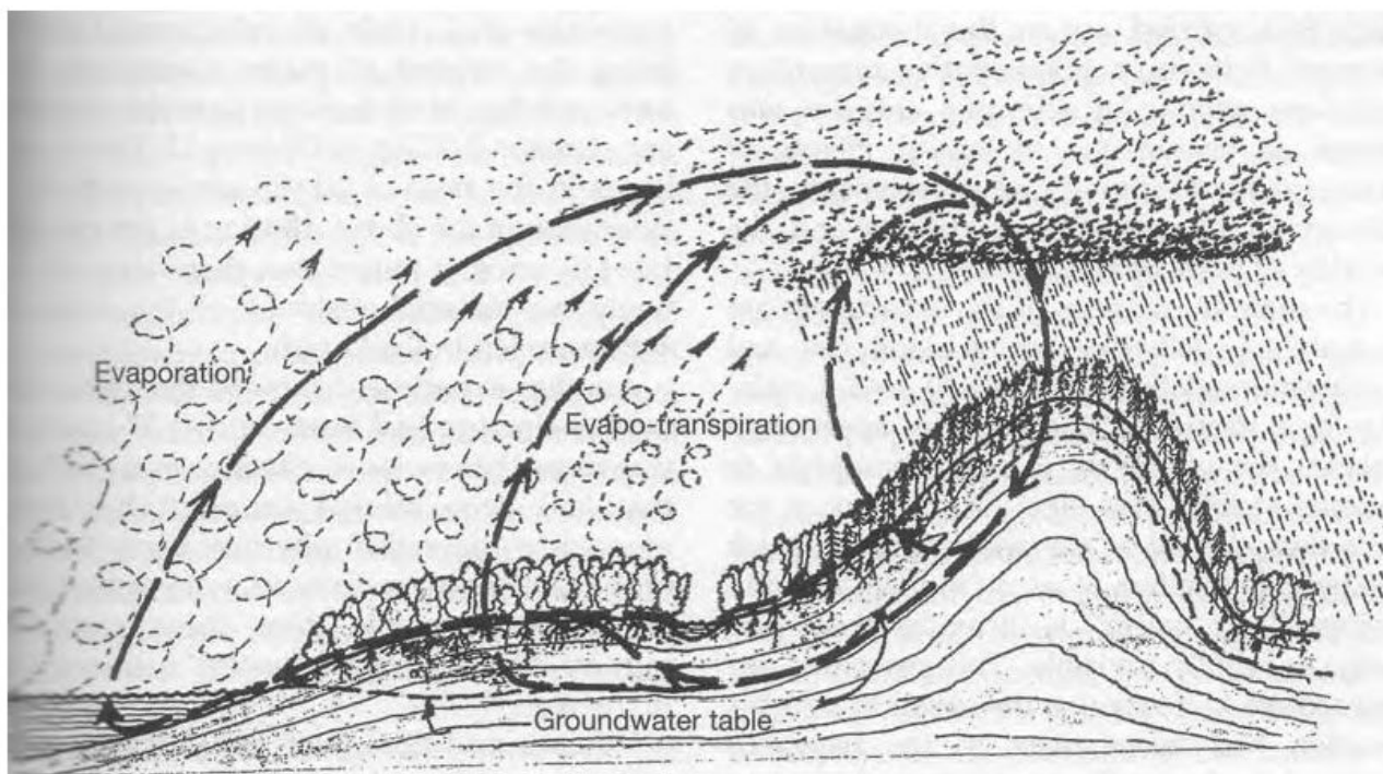
Рис. 9.1 полный гидрологический цикл
