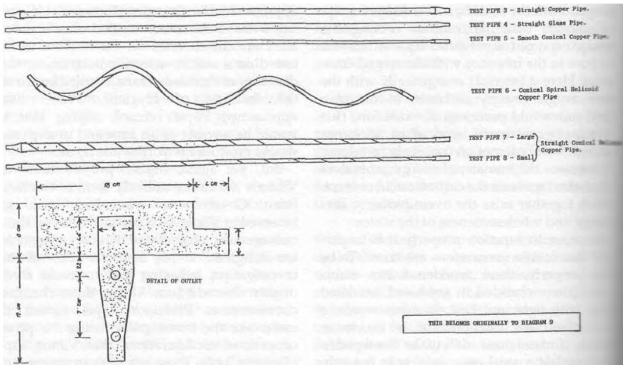
Рис. 14.5 трубы различной конфигурации, которые Шаубергер представлял проф. Попелью
