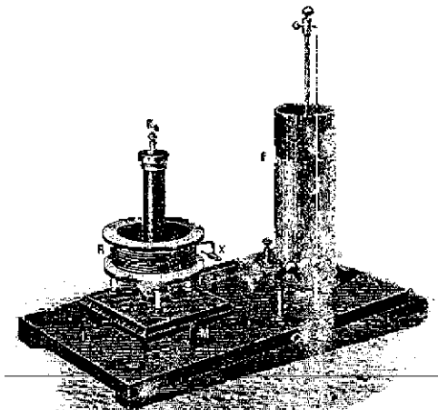
Рис. 454. Прибор для опытов Тесла
