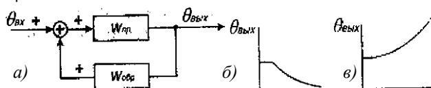
Рис. 4. Энергетическая установка, охваченная положительной обратной связью: а) структура; б) затухающий переходной процесс; в) расходящийся переходной процесс.
